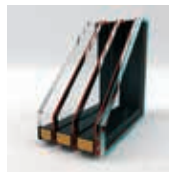
VERGLASUNG U8 U_g = 0,3 \text{ W/m}^2\text{K}
