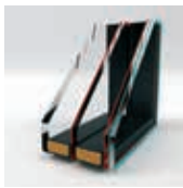
VERGLASUNG U6 U_g = 0,5 \text{ W/m}^2\text{K}
