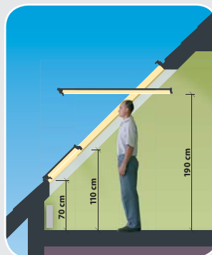
Fenster mit höher versetzter Schwingachse und unterem Festelement
