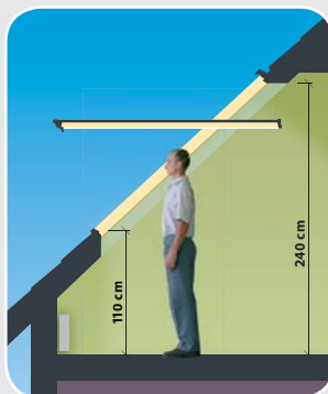
Fenster mit höher versetzter Schwingachse
