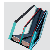
VERGLASUNG U6 Ug = 0,5 W/m²K
