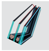
VERGLASUNG P5 Ug = 0,5 W/m²K
